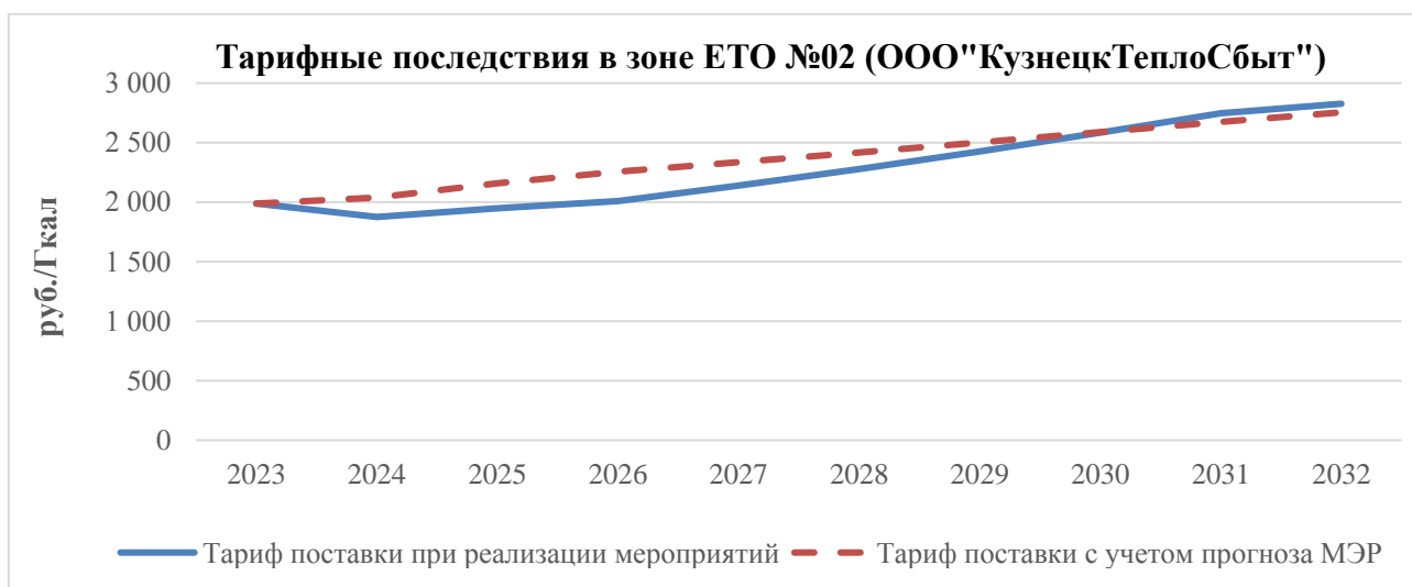
Рисунок 4.2 – Прогноз тарифа ООО «КТС» на тепловую энергию для потребителей
