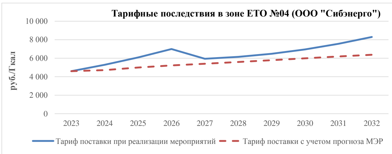
Рисунок 4.4 – Прогноз тарифа ООО «СибЭнерго» на тепловую энергию для потребителей
